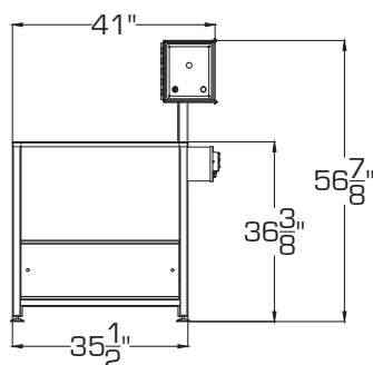
WNW 300
