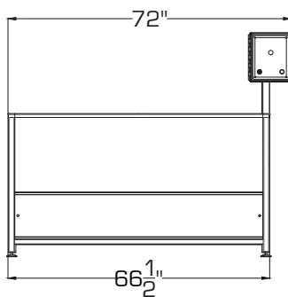
WNW 600
